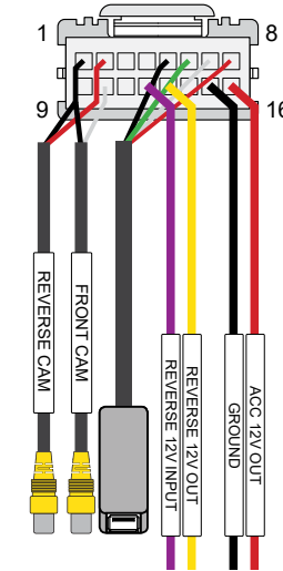
AV CABLE
